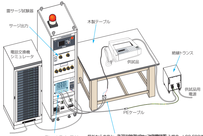
屋外からの非シールド対称信号線への試験を行う場合、LSS-F03では試験器の設定の変更を行うことで試験を行うことができます。
