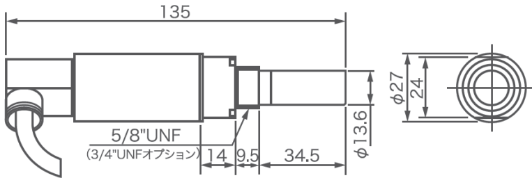
TK-100 露点トランスミッター
