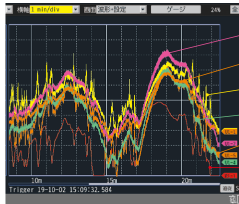
自動車のボディフレームにひずみゲージ貼付けて測定。走行中の車速と振動波形の例
