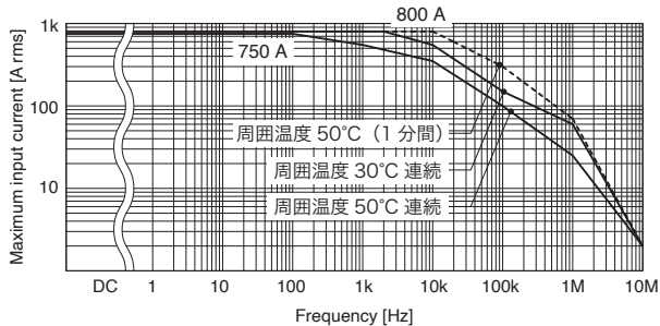
周波数ディレーティング
