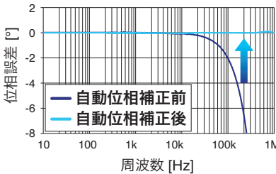
AC/DC カレントセンサ CT6904A の位相特性の補正例 (代表値)
