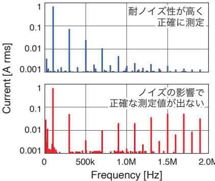
上：CT6904A CMRR 120 dB 以上 (100 Hz) 下：CMRR の低いセンサー
