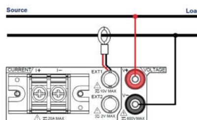
2系統の外部電流センサー入力
