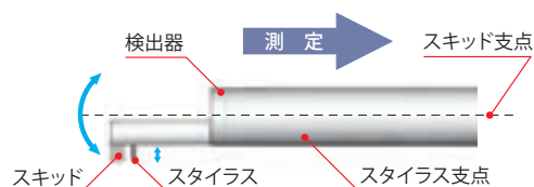
スキッドによる段差測定例
