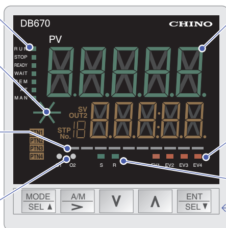
DB670前面部
