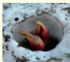
雪を融かしながら発熱しているザゼンソウ (岩手大学撮影)
