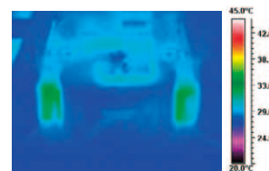
DC30A/10 分間入力時の 温度分布イメージ
