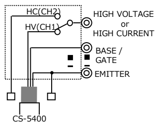
CS-710回路イメージ
