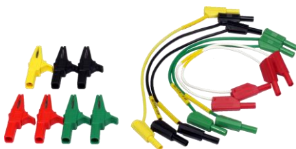
標準リードセット CS-005 (CS-3100を除く全機種標準添付) バナナケーブル 30cm (HV用赤2本、緑2本、黒2本、黄1本) ワニ口 (赤2個、緑2個、黒2個、黄1個)
