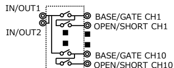
ゲート/ショートユニット CS-707 カーブトレサ側: 300V/7.5A/15A(Pulse) デバイス側: 5kV/7.5A/15A(Pulse) 10CH
