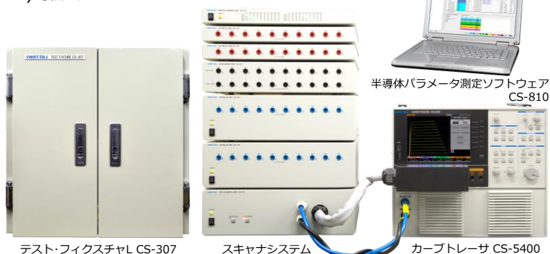
テスト・フィクスチャL CS-307
