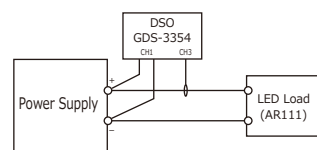
オシロスコープ GDS-3354 を使用しての LED 動作実験
