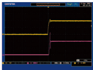
CV 優先モード：LED 順電圧 V_f にて突入電流とサージ電圧が発生
