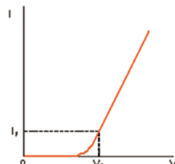
ダイオード V_f 特性
