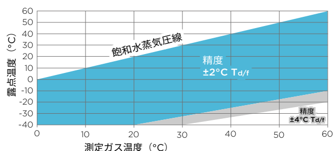
露点精度と計測条件との関係 (DMP80A)
