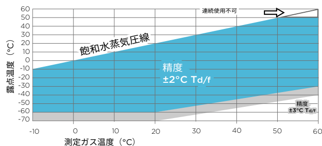
露点精度と計測条件との関係 (DMP80B)
