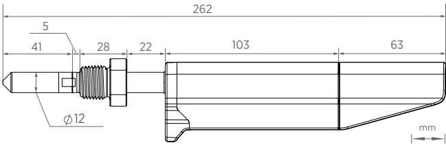
NPT1/2"ネジ付きDMP80シリーズ プローブの寸法
