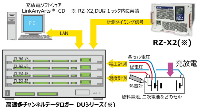
充放電ソフトウェア、データロガーとRZ-X2の構成イメージ
