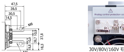
30V/80V/160V モデル出力端子 バスバー形状
