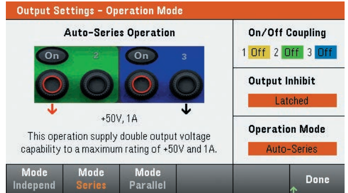
図3. 出力電圧を2倍にする自動直列動作
