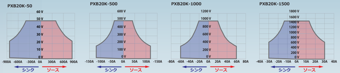
【動作領域概念図】
