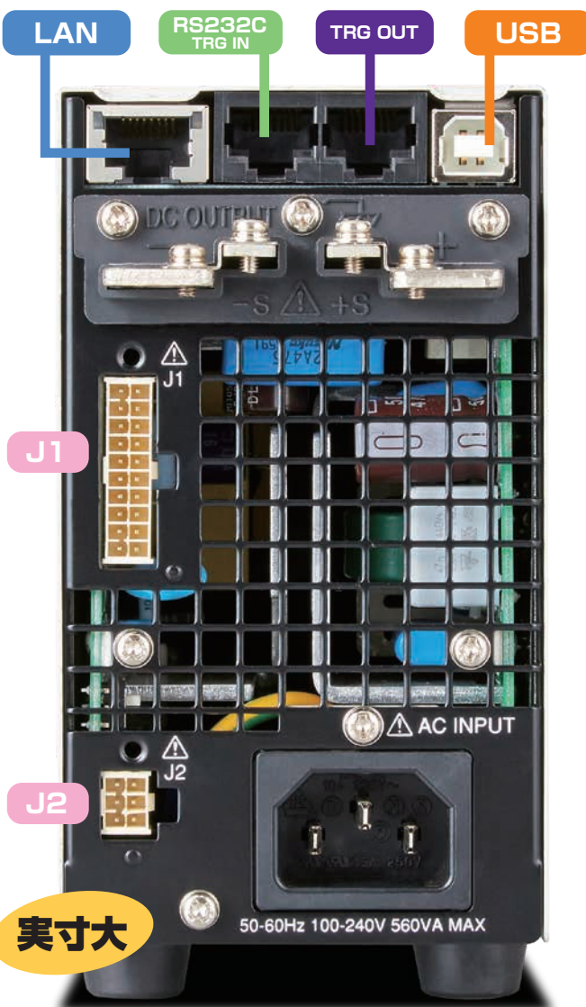
リアパネル：400W モデル
